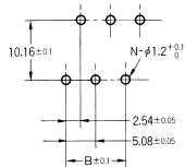
印刷基板加工尺寸 (BOTTOM VIEW)
