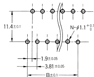
印刷基板加工尺寸 (BOTTOM VIEW)
