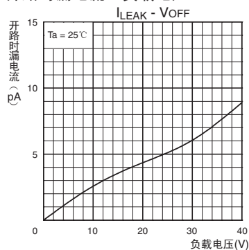
开路时漏电流—负载电压
